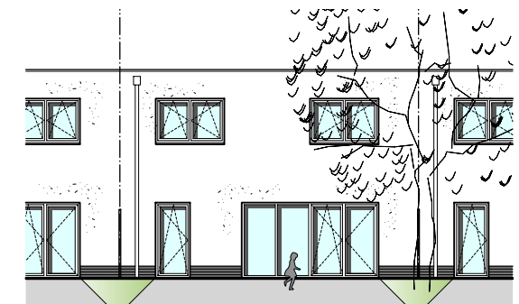
Gartenansicht
